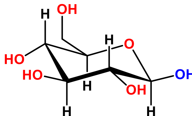
\beta -D-glukopiranoza
