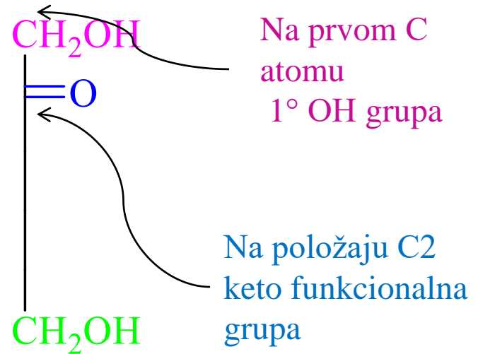
ketoze
