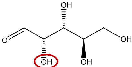
D-arabinose
