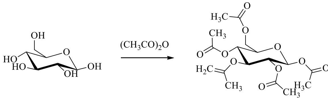
Pentaacetat glukoze
