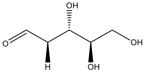
D-deoxyribose
